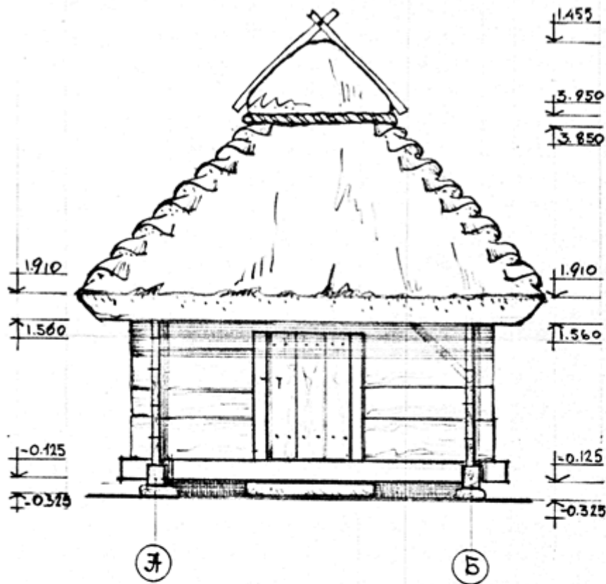
Національний музей народної архітектури та побуту України Експозиція «Середня Наддніпрянина» Комора с.Молодецьке. Фасад 1
