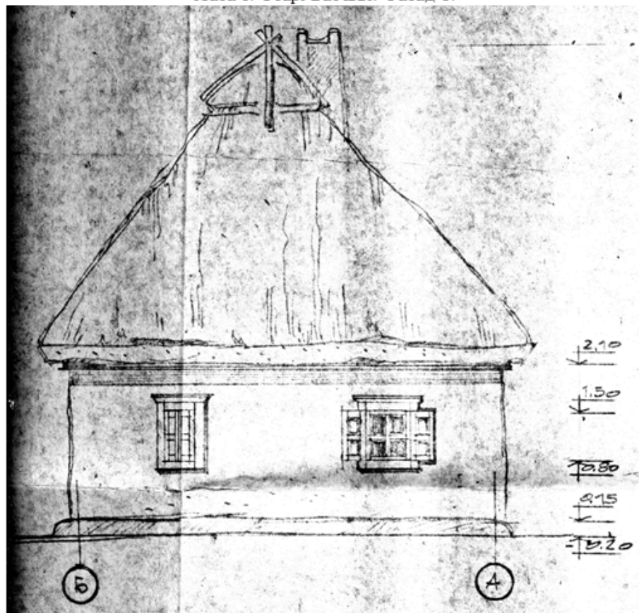
Хата с. Старі Бабани. Фасад 2
