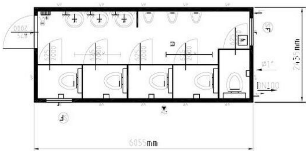
Схематичний план громадської вбиральні модульного типу
