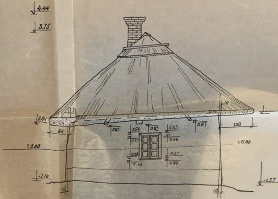
Фасад "Б" М 1:50
