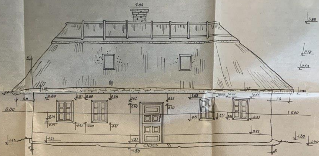
Фасад „А“ М 1:50
