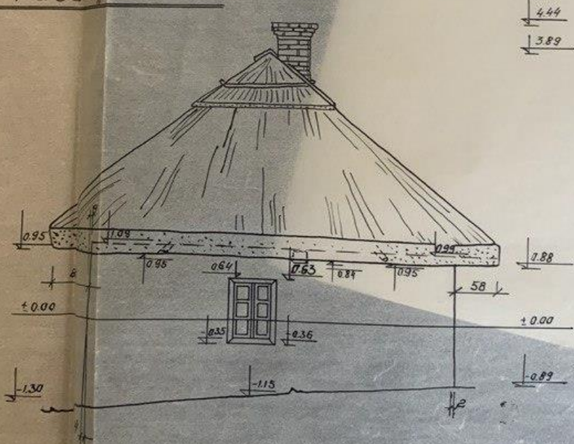
Фасад "Г" М 1:50
