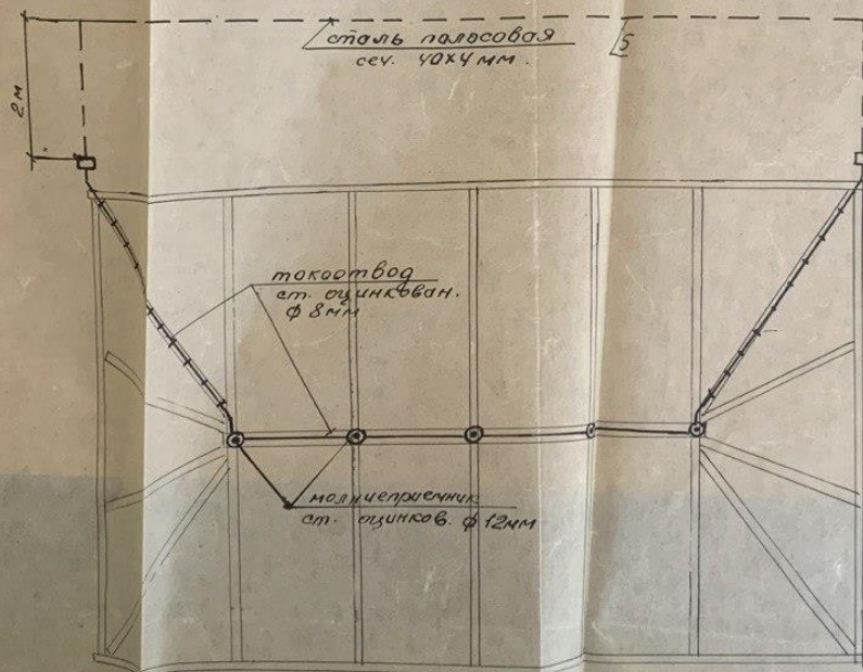
План кровли
