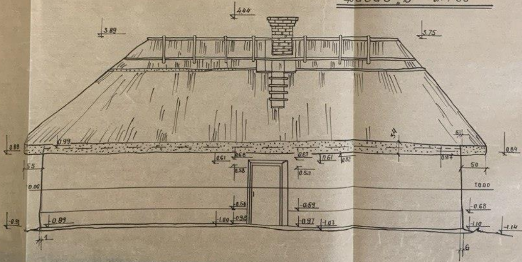
Фасад „Б“ М 1:50
