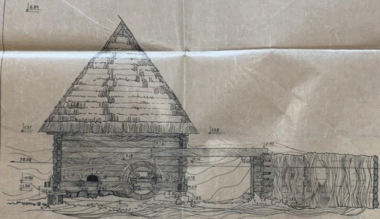
ПІВНІЧНО ЗАХІДНИЙ ФАСАД М 1:50
