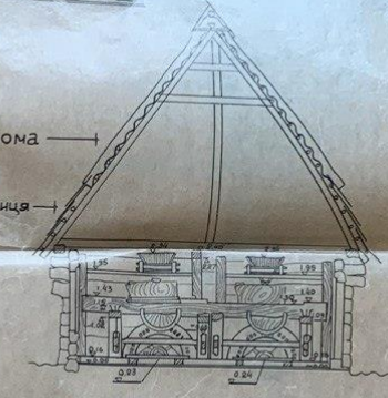
Розтин V-V М 1:50
