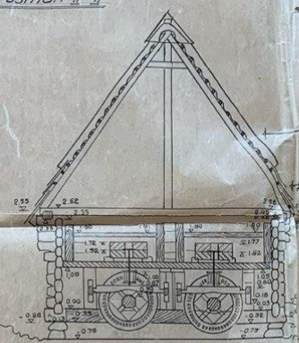
Розтин IV-IV М 1:50
