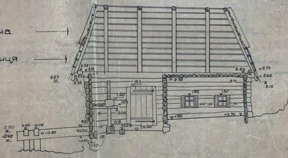
Розтин IV-IV М 1:50
