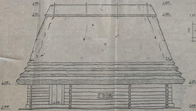
ФАСАД III М 1:50
