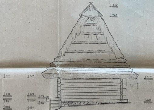
ФАСАД II М 1:50
