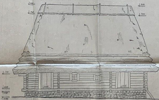
ФАСАД III М 1:50
