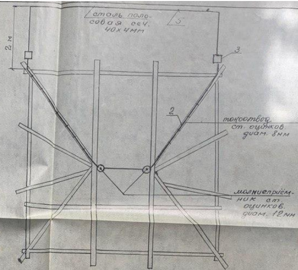
План кровли.
