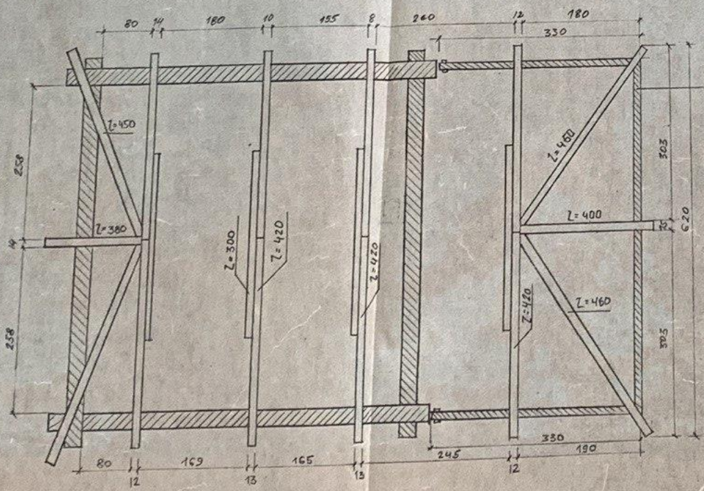
ПЛАН КРОКВ М 1:50
